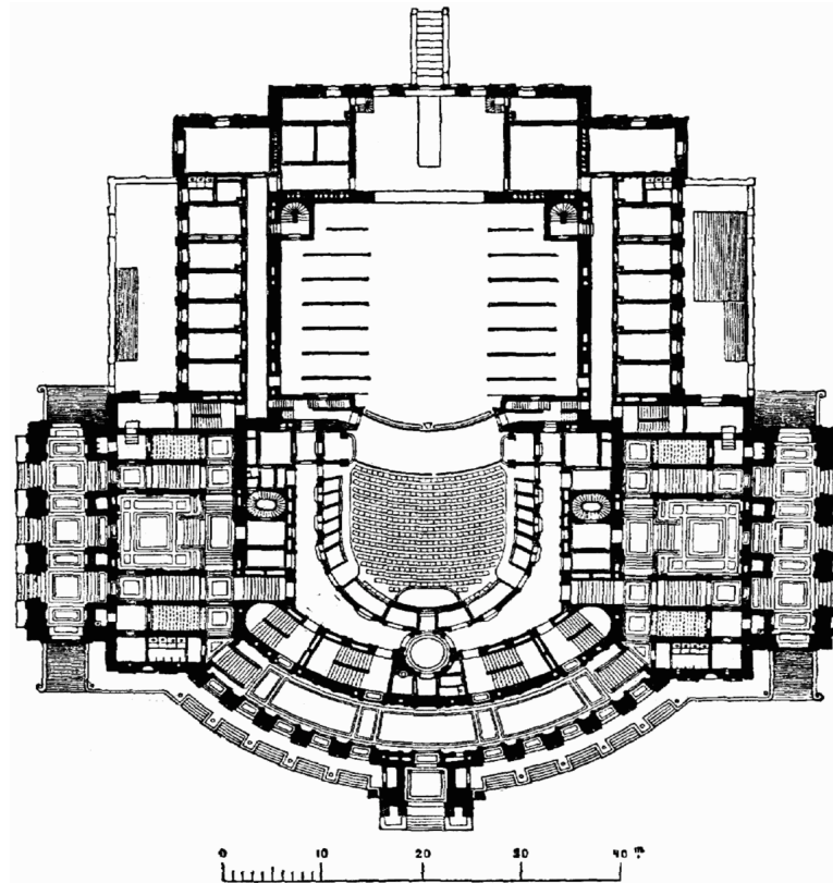
Fig. 2. Neues Hoftheater zu Dresden (Arch. G. Semper). Grundriß in Parketthöhe.
